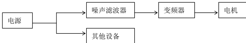
电源侧噪声滤波器的设置
